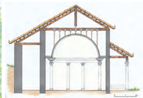
SEZIONE
